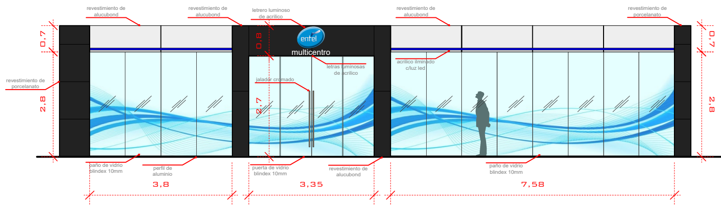
Facha Frontal
